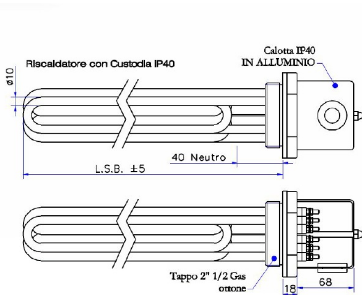
Riscaldatori su tappo 2" ½ gas in ottone 3 Elementi Ø10 mm. ad OCCHIELLO Terminali: Acc. carbonio Dadi e rondelle: ottone
